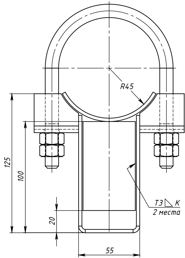
Поз.3 (Ложемент)
