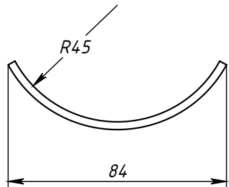
Поз.5 (Хомут)
