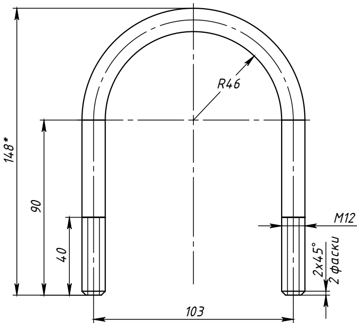
Поз.5 (Хомут)
